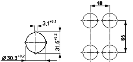
Bohrung für Bedienelemente Drilling for actuator elements Perçage pour éléments de commande Minimale Abstände der Bohrungen Minimum clearances between drillings Distance minimale des perçages
